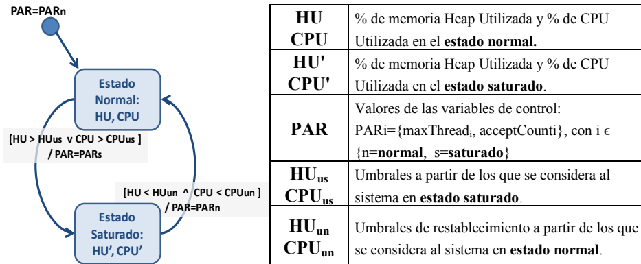
Fig. 6. Máquina de Estados para la estrategia de control aplicada.
