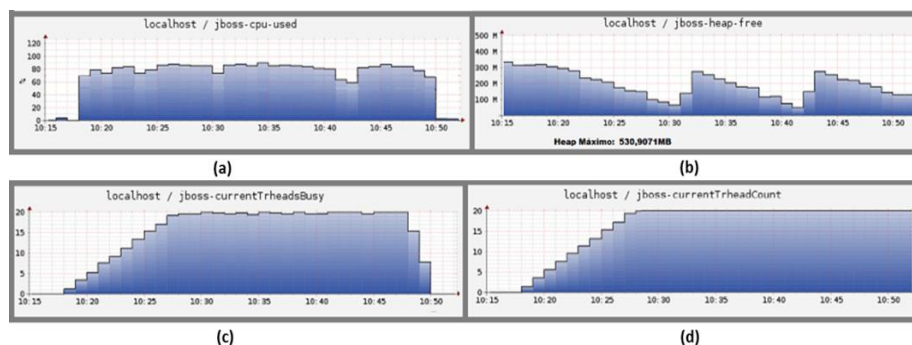
Fig. 9. Caso de Test 0 (ejecución sin DECSS). (a) Consumo de CPU (b) Memoria Heap libre (c) Cantidad de threads ocupados (d) Cantidad de threads creados.
