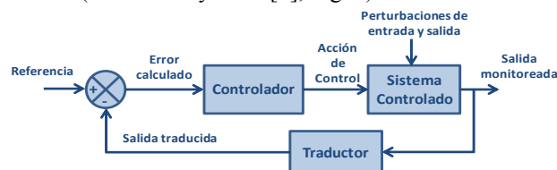
Fig. 1. Diagrama en bloques de un lazo de control a lazo cerrado.
